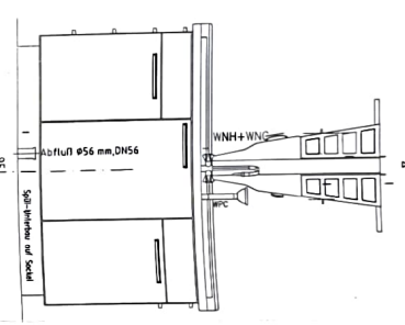
Auf Tischchasse Ansicht 3
