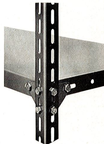
Eingeschraubter Stahlboden mit Eckplatten
