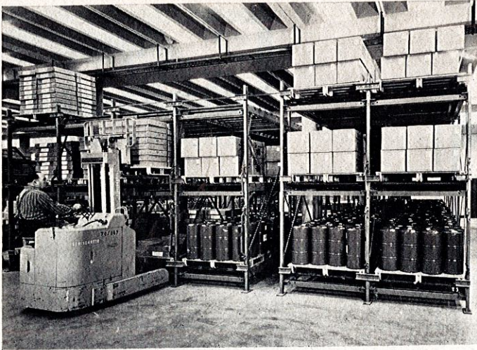
Fließlager zwischen Fertigung und Versand mit KIND Stahl-Durchlaufregalen nach dem Prinzip "first in – first out".
